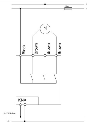
Anschlussbeispiel AKK-03UP.03 Fancoil
