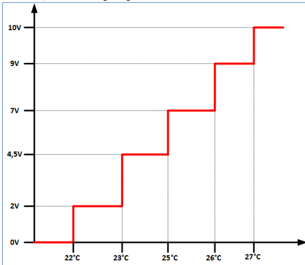
Abbildung 19: Stellwertvorgabe über 2 Byte Gleitkommawerte als Stufenschalter
