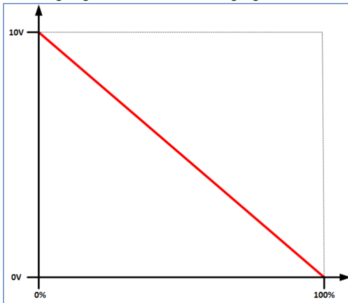
Abbildung 22: invertierter Wirksinn
