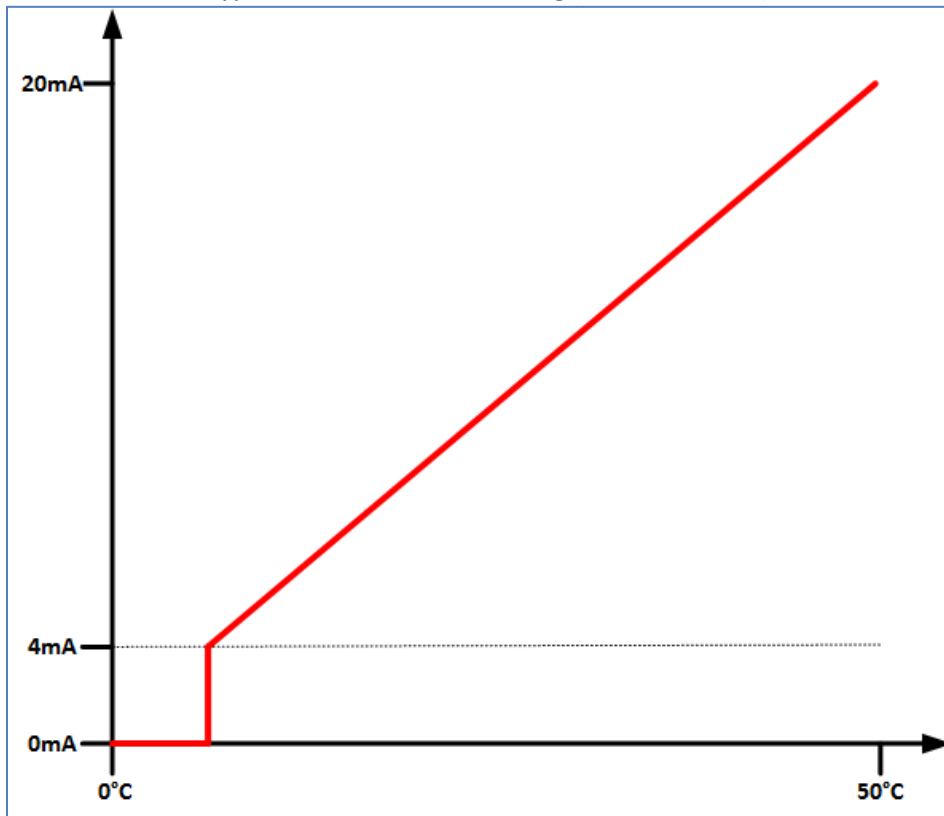
Abbildung 10: Grafik Messwertskalierung 2
