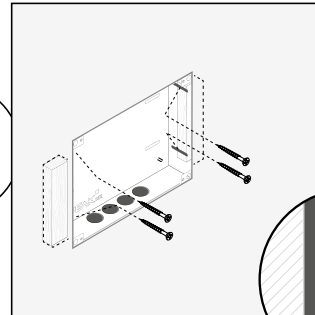
Beide Holzklötze in der Wand befestigen. Fit the two wooden fillets inside the wall.
