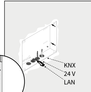
Bündig zur Wand Box flush with wall
